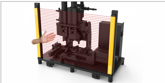
安全光幕应用案例
