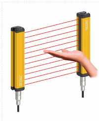
光轴间距 (20mm)
